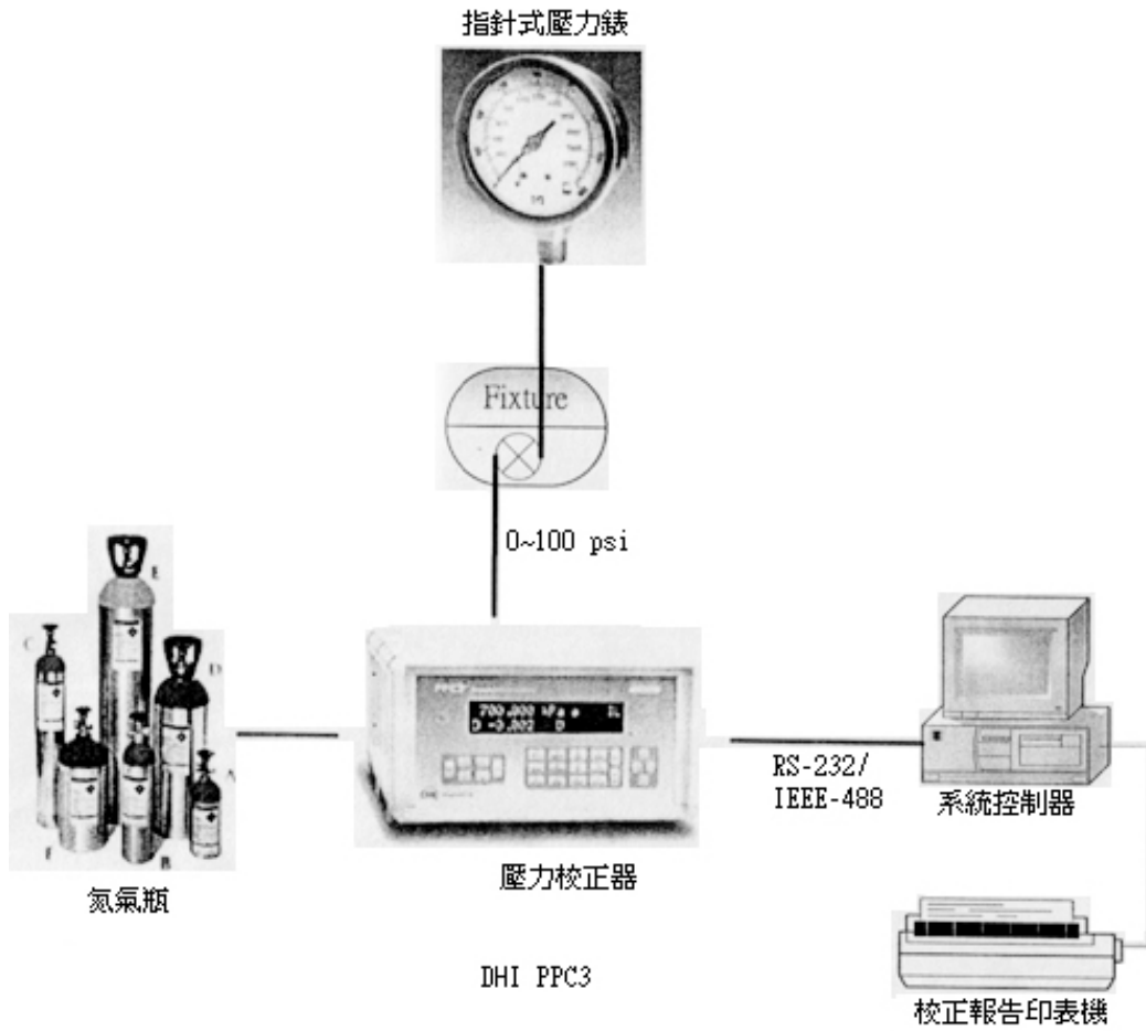
指針式壓力錶校正系統
