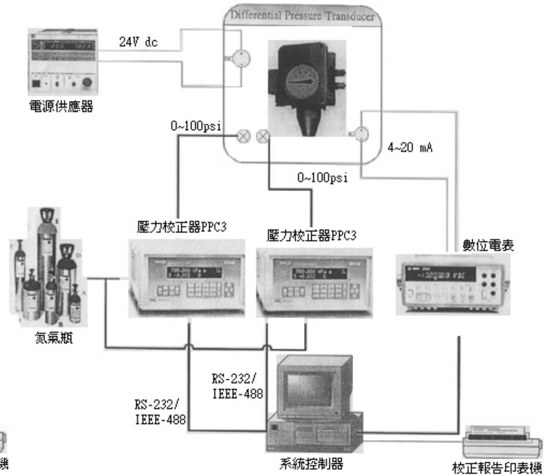
差壓傳送器校正系統
