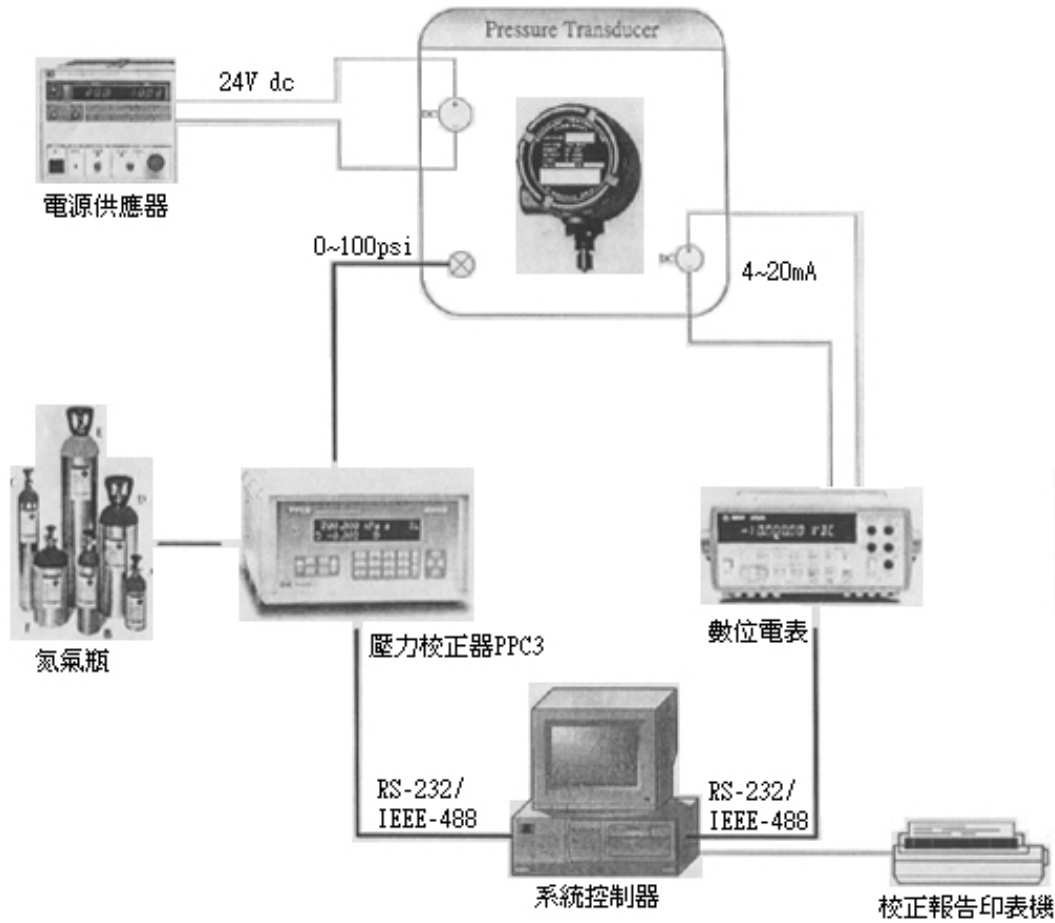
壓力傳送器校正系統
