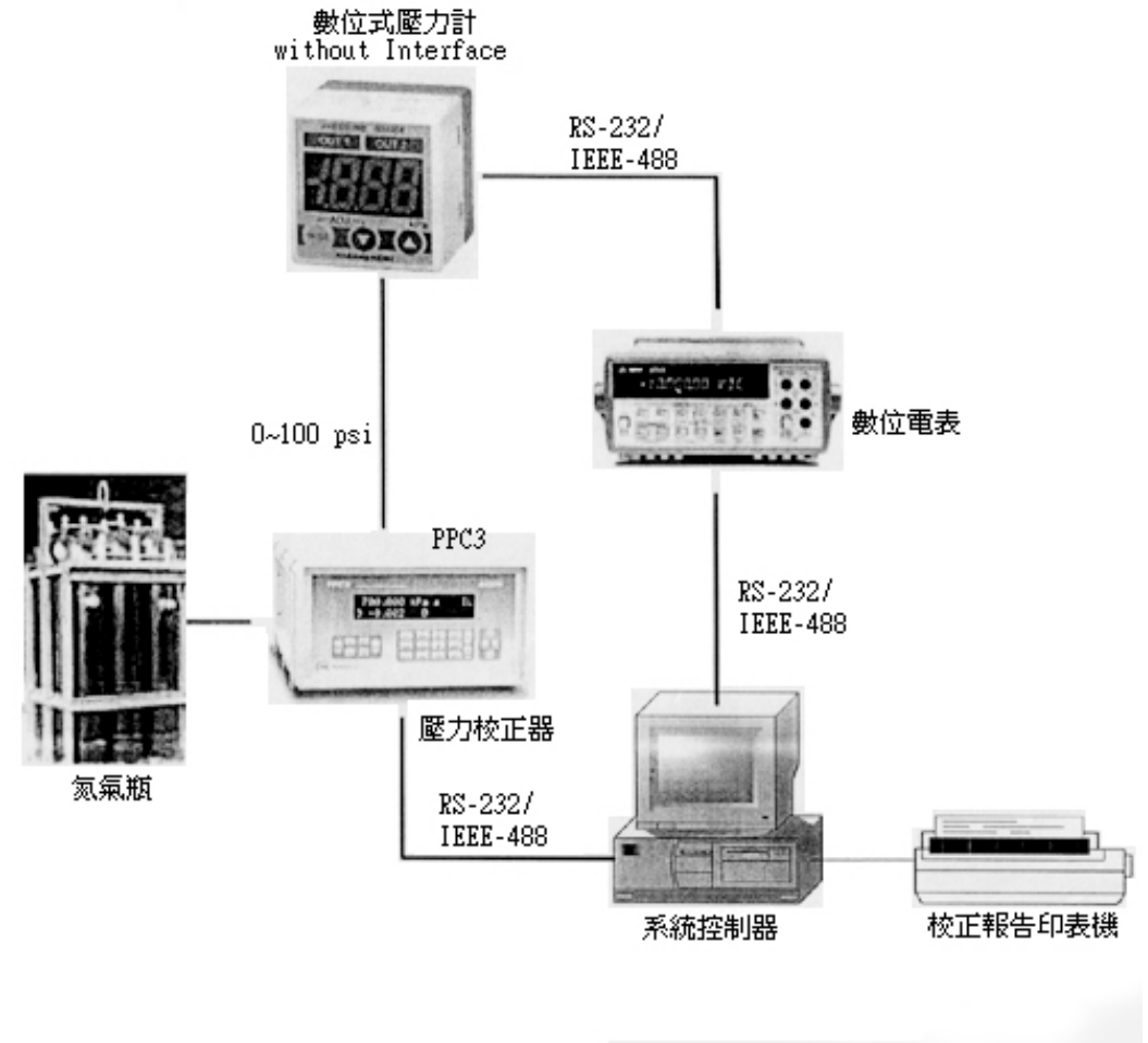
數位式壓力錶校正系統
